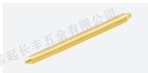
CFCZ-004 类别: 插针系列 名称: 插针端子 尺寸: \Phi 1.3 \times 17 材质: 铜材H59
