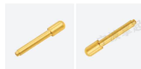
CFCZ-015 类别: 插针系列 名称: 插针端子 尺寸: \Phi 4.8 \times 27 材质: 铜材H59
