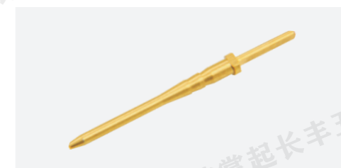
CFCZ-016 类别: 插针系列 名称: 插针端子 尺寸: \Phi 3 \times 35 材质: 铜材H59
