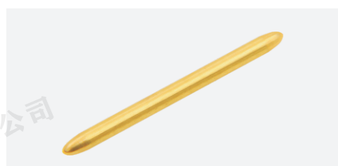
CFCZ-005 类别: 插针系列 名称: 插针端子 尺寸: \Phi 1.3 \times 17 导弹头 材质: 铜材H59
