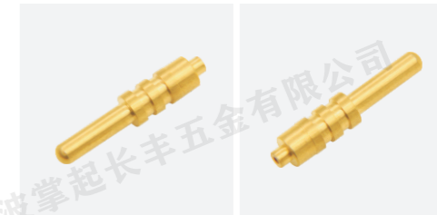
CFCZ-012 类别: 插针系列 名称: 插针端子 尺寸: \Phi 3 \times 20 材质: 铜材H59
